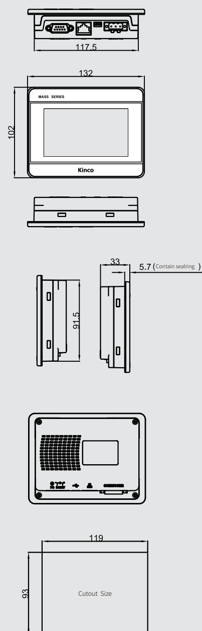
Dimension(Unit:mm)
